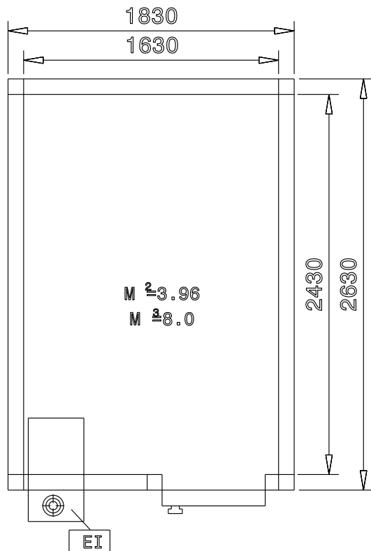
Zij aanzicht
